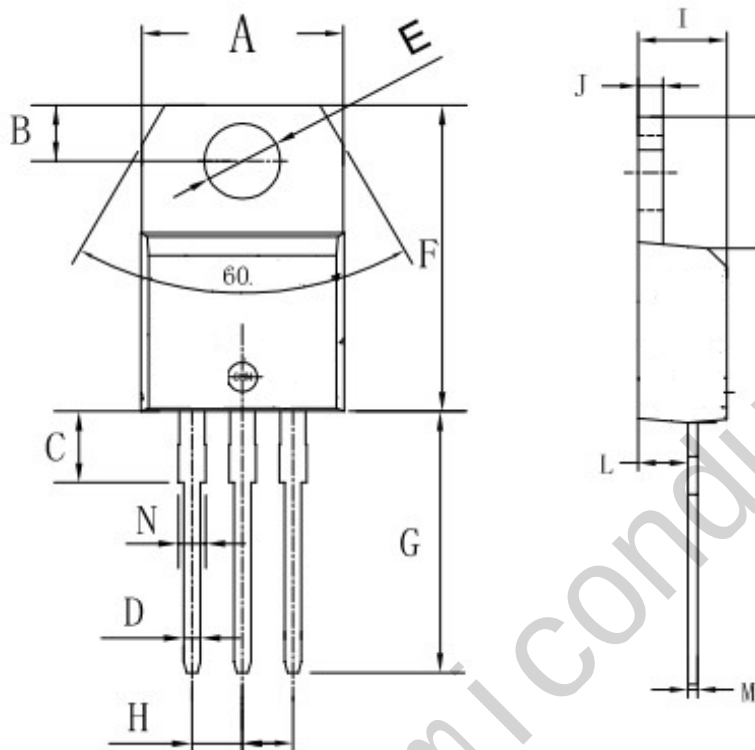
外形尺寸图 / Package Dimensions
